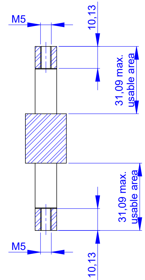
CUT A-A
